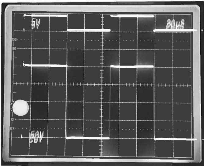
NON INVERTING
